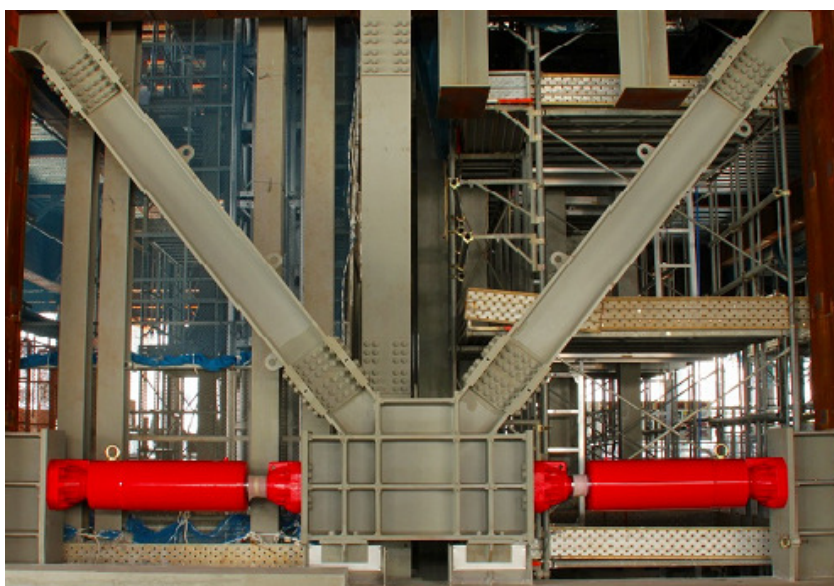
BDH2000型オイルダンパ
