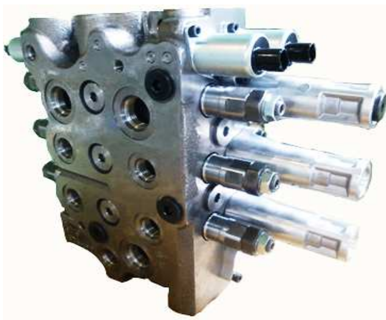
コンパクトトラックローダ用コントロールバルブ(KVML-120)
