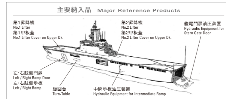
輸送艦「おおすみ」 Tank Landing Ship OSUMI
