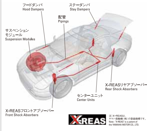
クルマに搭載されるショックアブソーバ(ダンパ)製品群 Automobile Shock Absorber (Damper) Product Group
