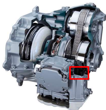
ジヤトコ株式会社様 CVT 外観
